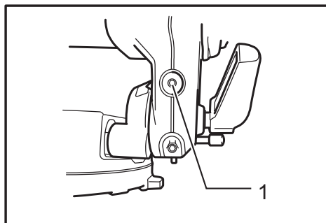
► 1. Boulon de réglage de l'angle de coupe en biseau 45° de gauche
