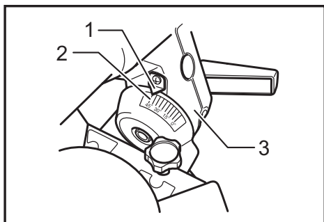
► 1. Apuntador o puntero 2. Escala de bisel 3. Brazo
