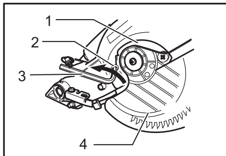
► 1. Couvercle central 2. Boulon hexagonal 3. Clé hexagonale 4. Capot de sécurité
