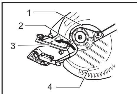
► 1. Cubierta central 2. Pernos de cabeza hexagonal 3. Llave hexagonal 4. Cubierta de seguridad
