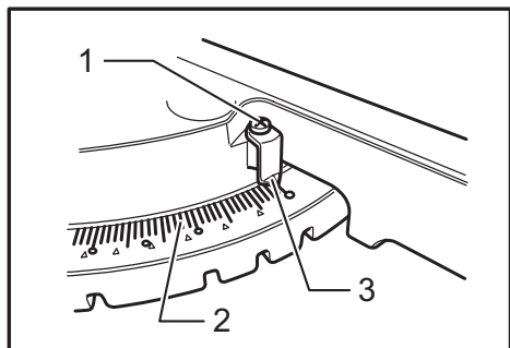
► 1. Vis 2. Échelle de coupe d'onglet 3. Index
